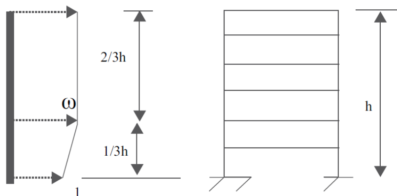
Figure 7 : Coefficient dynamique \omega
