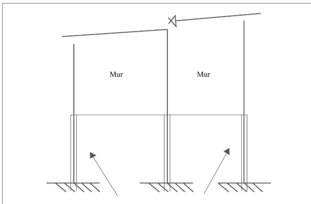
Figure 7.8 : Poteaux confinés sur toute la hauteur
