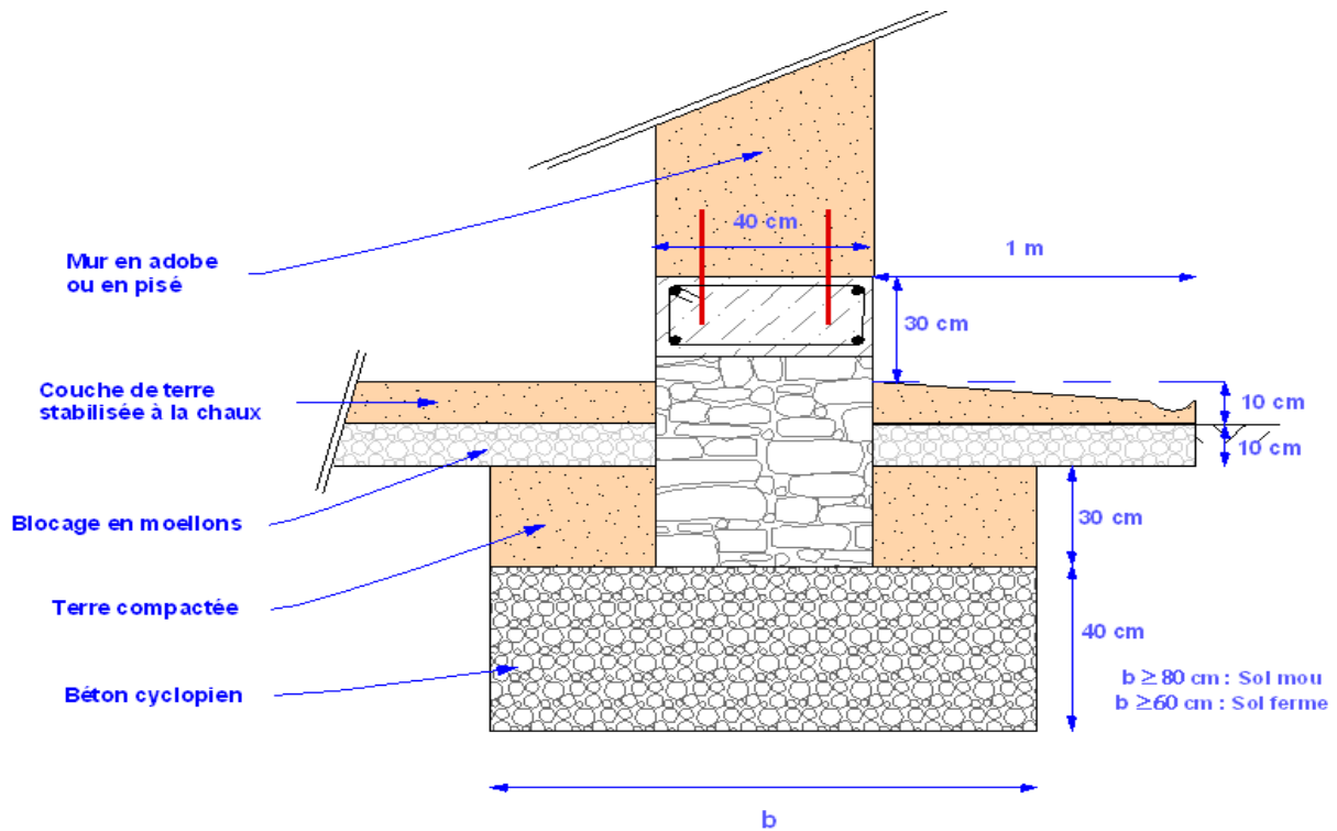
Fig.49. Fondation en béton cyclopéen + Chaînage en BA + Tiges d'attaches mur Chaînage
