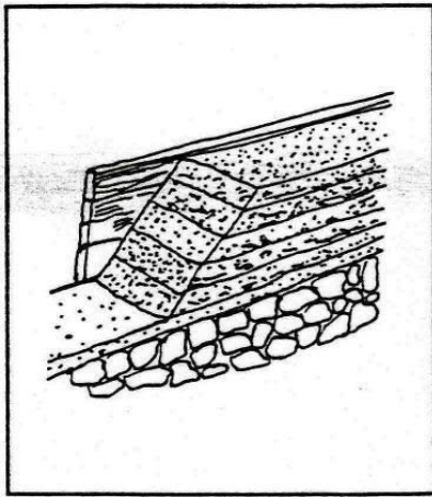
Figure n° 13 : Compactage par couche de terre
