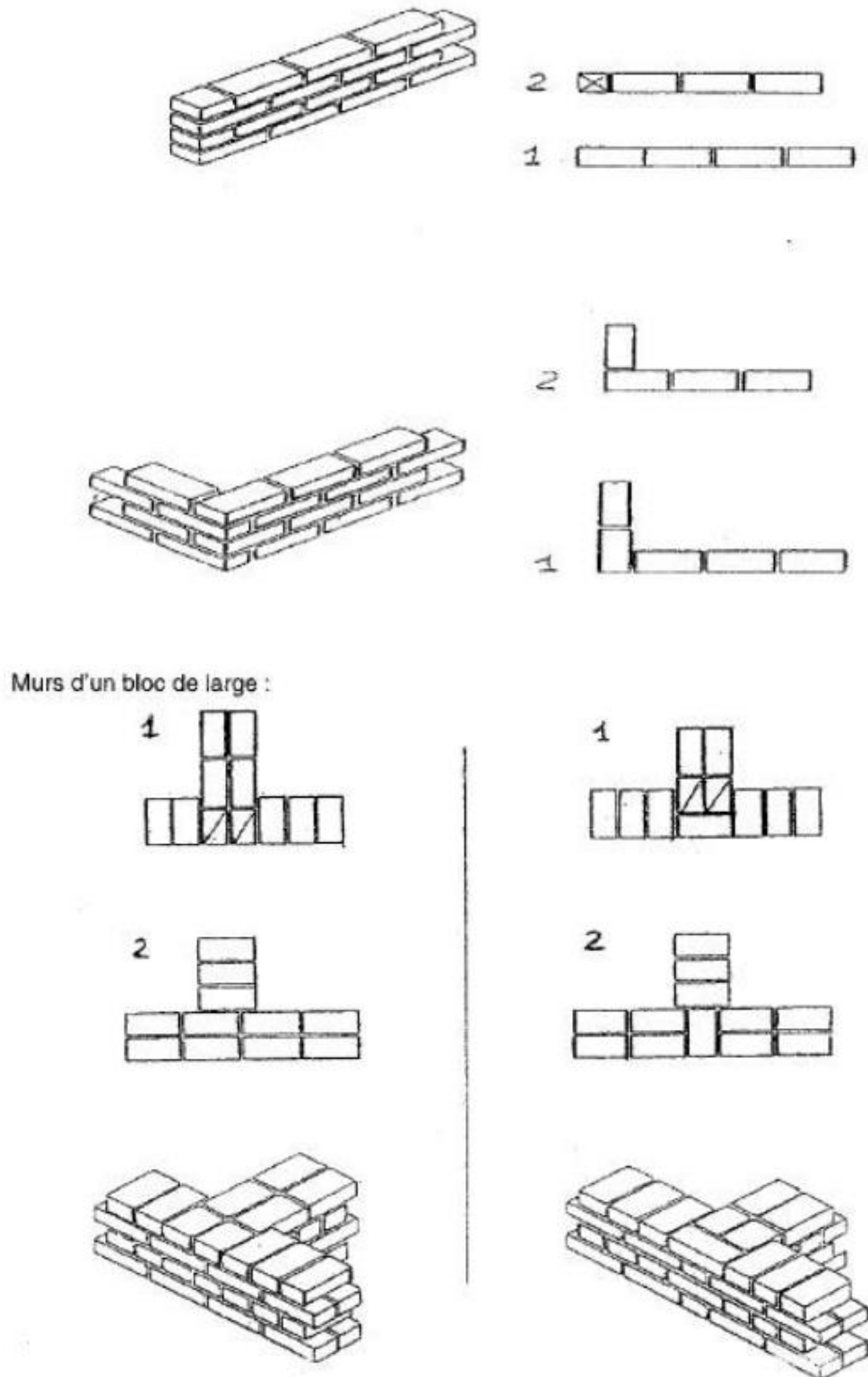
Figure n° 9 : Appareillage de base avec des blocs parallélépipédiques
