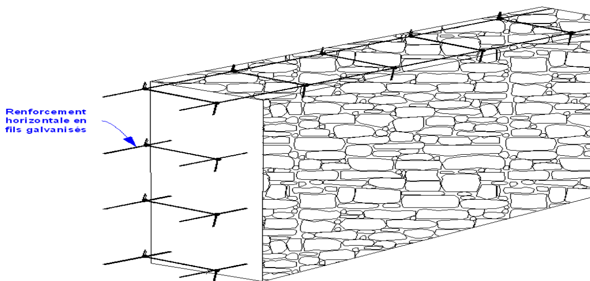
Fig.43. Renforcement horizontal par grillage en fils galvanisés
