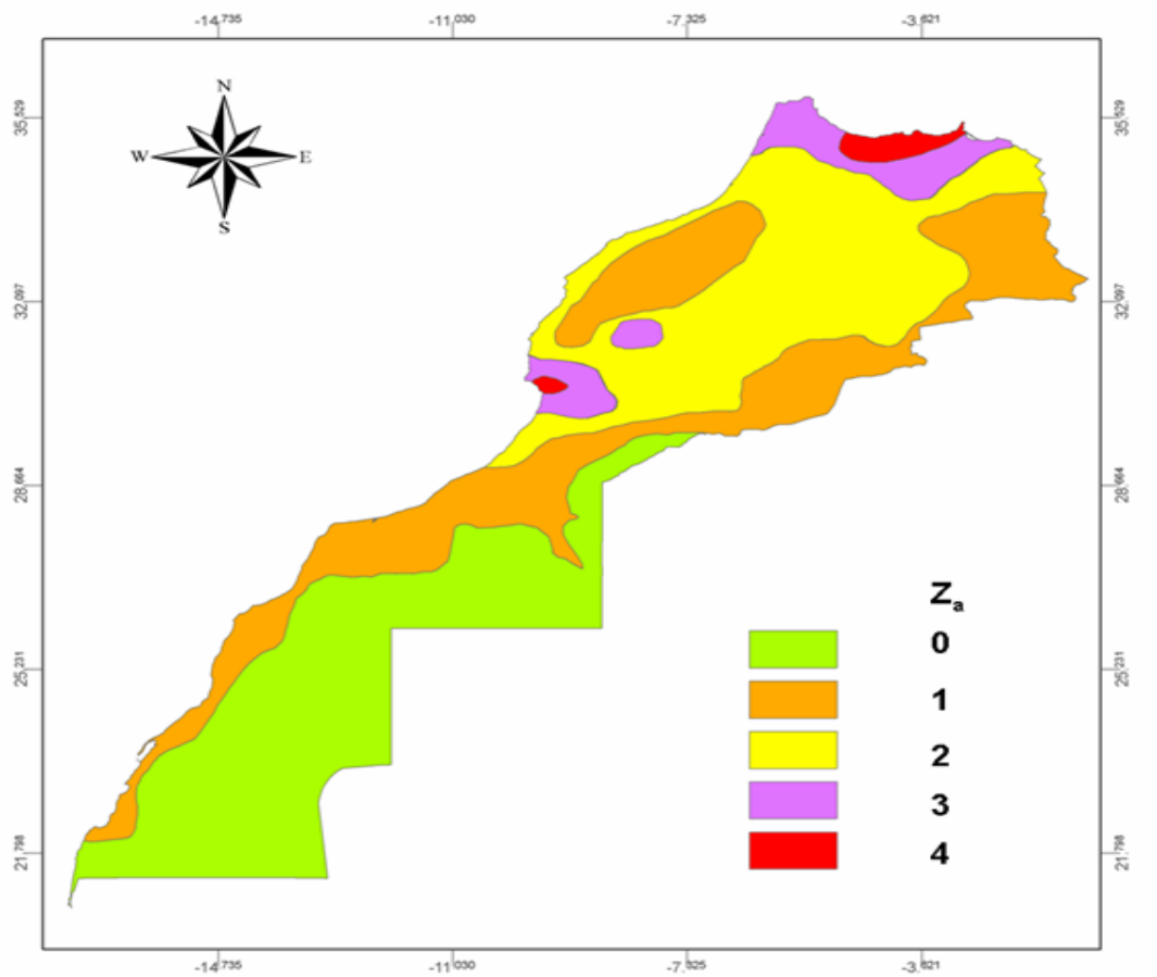
Fig.17. Zones d'accéléérations maximales du sol
