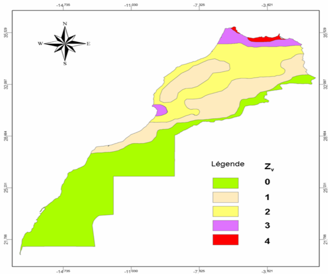
Fig.18 : Zones de vitesses maximales du sol
