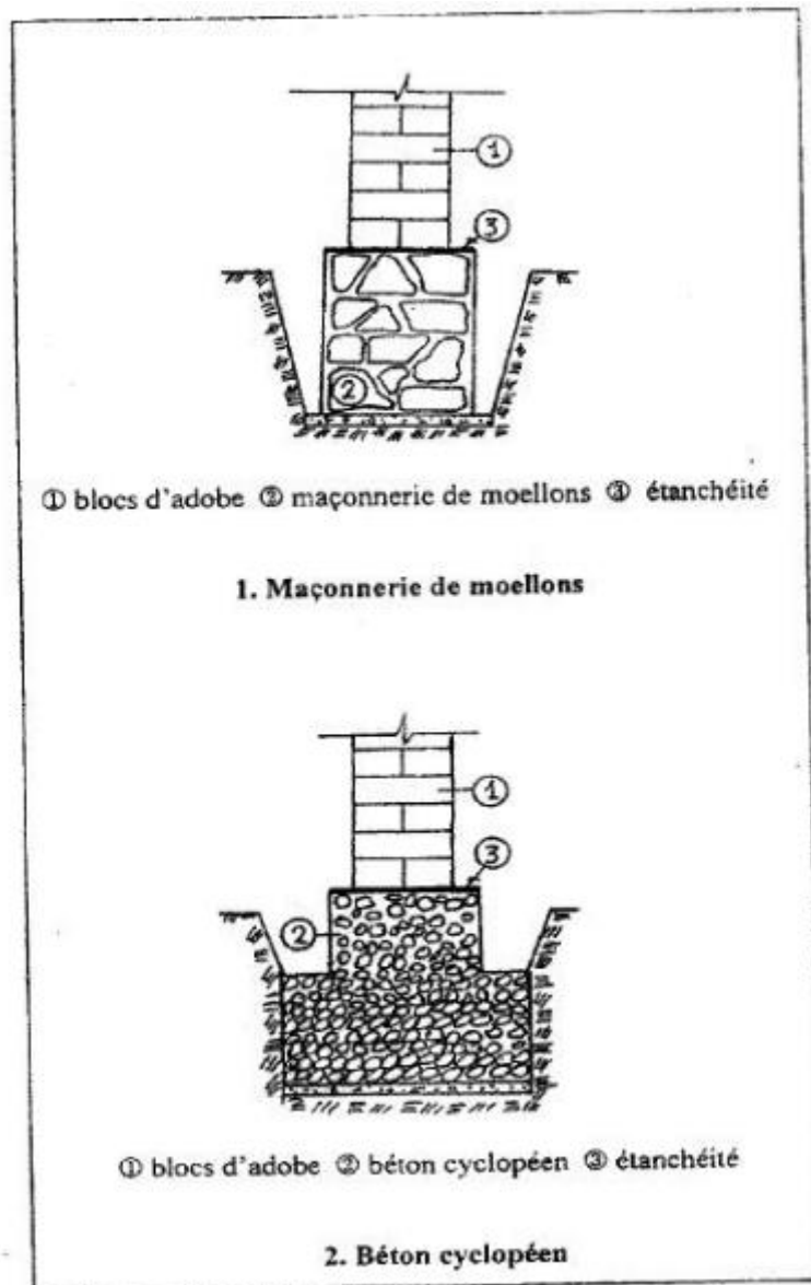
Figure n° 29 : Différents types de fondations (Adobe)
