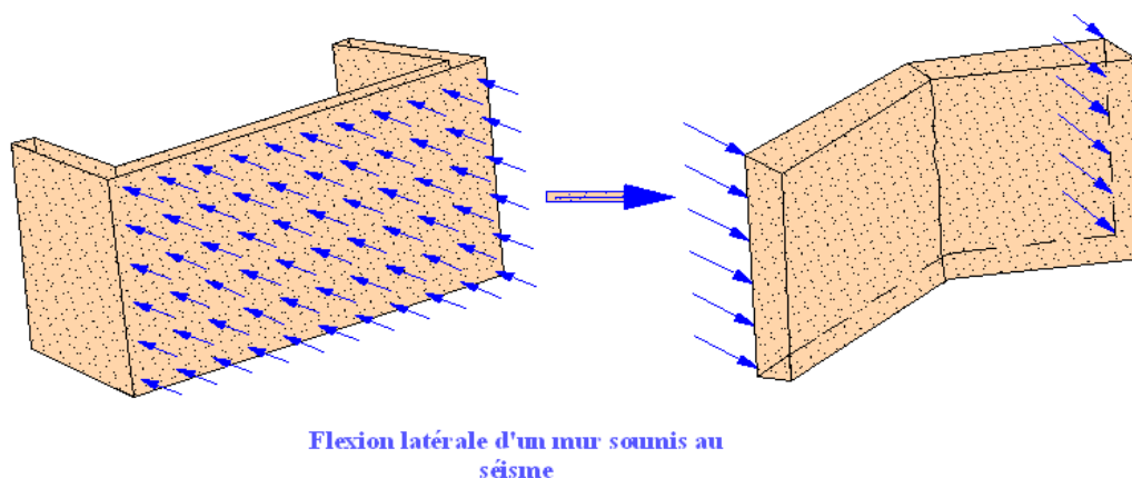
Fig.27. Flexion latérale d'un mur soumis au séisme
