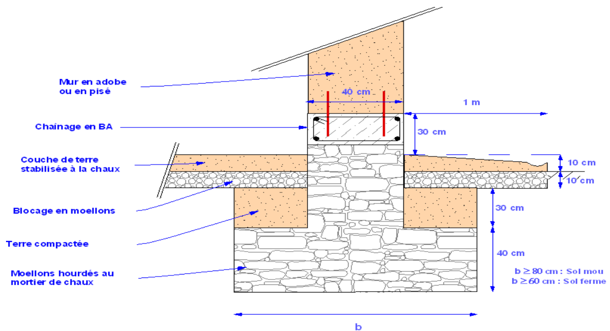
Fig.48. Fondation en maçonnerie de moellons + Chaînage en BA + Tiges d'attaches mur - Chaînage
