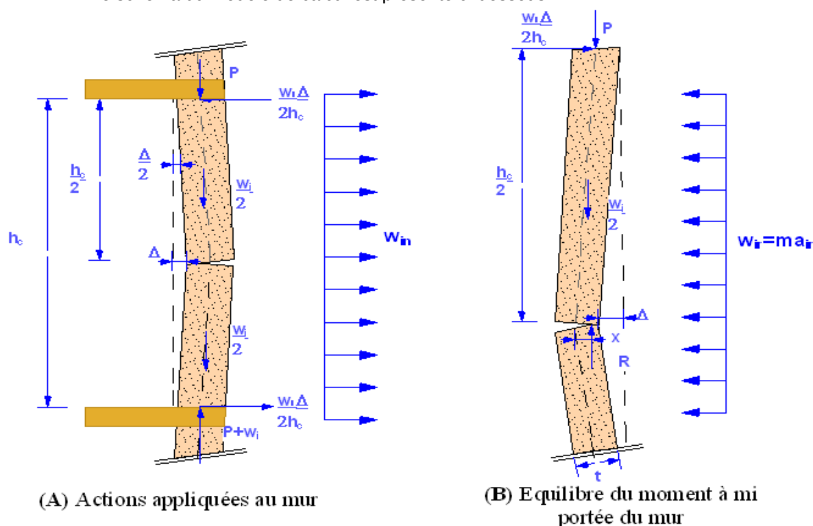
Fig.28. Schéma du modèle de calcul
