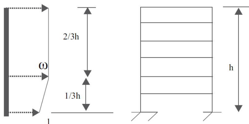
Figure 7 : Coefficient dynamique \omega
