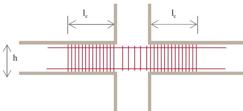
Figure 7.4 : Zone critiques d'une poutre
